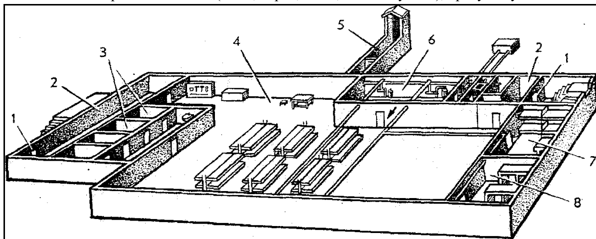
Рисунок 2.1 – План убежища
