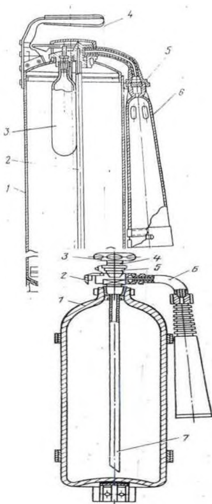
Рисунок 4 - Огнетушитель порошковый ОП - 10
