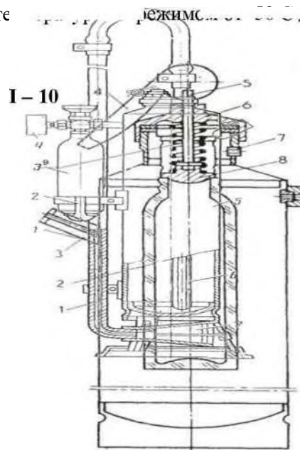
Рисунок 1 - Химический пенный огнетушитель
