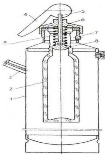
Рисунок 1 - Химический пенный огнетушитель ОХП - 10
