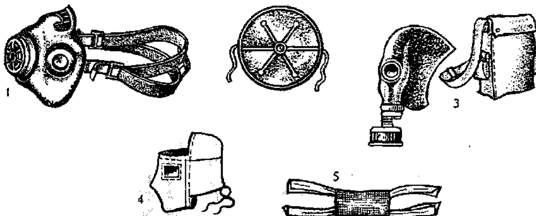
Рисунок 2.3 - Средства индивидуальной защиты органов дыхания 1 - респиратор Р-2; 2 - респиратор типа «Лепесток»; 3 - противогаз ГП-5; 4 - противопыльная тканевая маска ПТМ-1; 5 - ватно-марлевая повязка.
